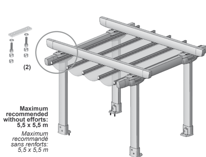
SET OF PERGOLA WITH REINFORCED CAPITALS KIT PERGOLA AVEC CHAPITEAUX RENFORCÉS
